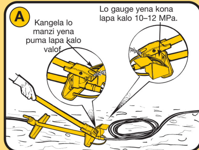
A. Lo mapomp yena setiwa skat yena enziwa mar lo ndawo yena setiwa lapa kayena yena funa setshiwa zonke skat. Kanjani: Faka lo gauge lapa kalo nozel kalo ntambu kalo pomp yena pelela. Futi wena pompa lo pomp kalo sandla.
